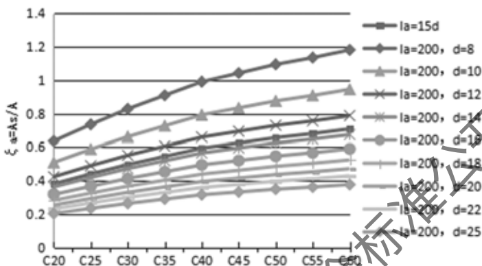
图 A-1 带肋钢筋 (HRB400) l_a = 15d 和 l_a = 200mm 时的 \xi_a = A_s/A 曲线图
