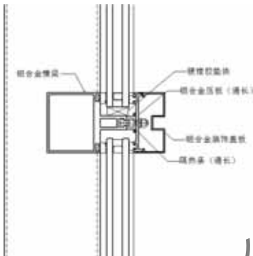
图 6-1 明框托条构造示意
