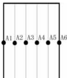
图 11-2 单索幕墙与周边支承结构立面示意图
