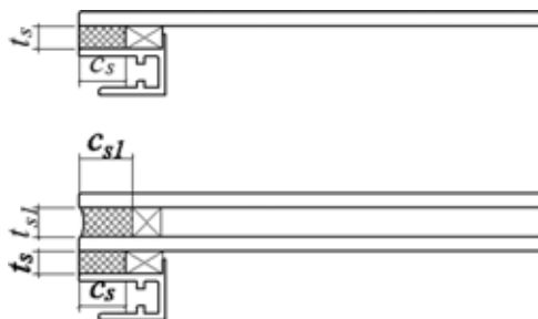
图 6.2.19 隐框玻璃板块结构胶尺寸及位置配合示意图
