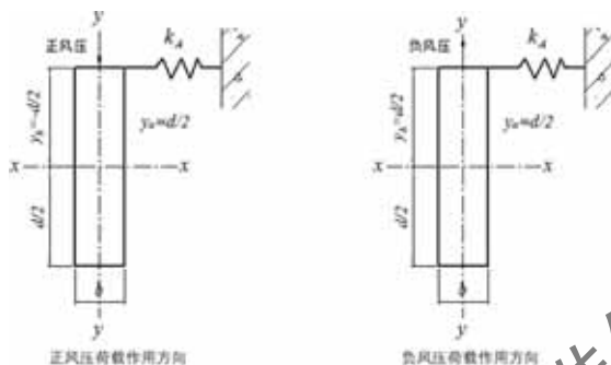
图 10-1 不同荷载作用方向玻璃肋稳定计算
