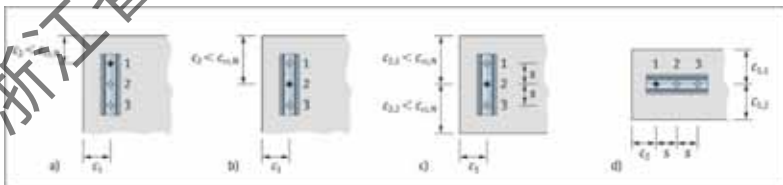
图 B. 3. 8 槽式预埋件边角距离 c_2 取值示意图
