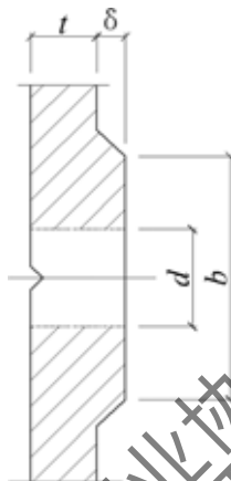
图 7-1 局部加厚简图
