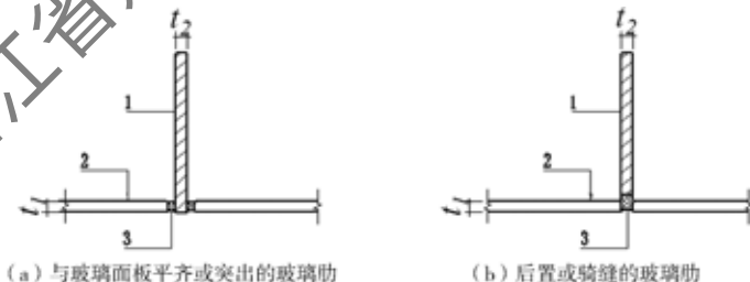
图 10.3.9 全玻璃幕墙玻璃肋示意图
