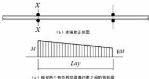
图 10-2 间隔的玻璃肋侧向约束
