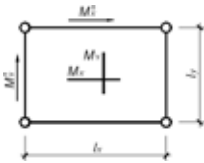
图 C.2.1 四角支承板的计算简图
