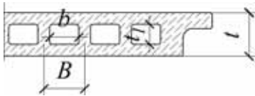
图 6-6 30mm 厚陶土板构造示意图
