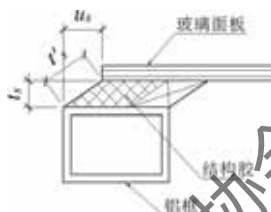
图 5-2 结构胶剪切应变示意图
