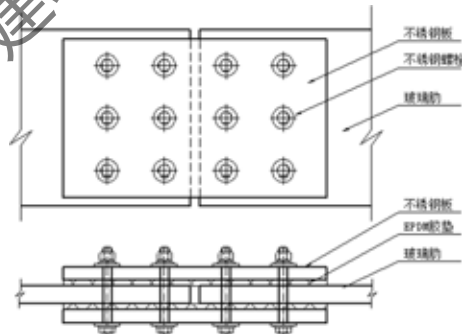
图 10 - 4 玻璃肋机械连接示意图
