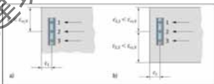
图 B.4.6 槽式预埋件锚筋受边角影响示意图 a) 受一个角影响；b) 受 2 个角影响
