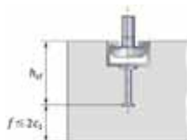
图 B. 3. 11 槽式埋件在较薄的混凝土基材中
