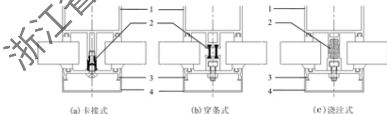
图 G.1.2 明框构件式幕墙隔热方式
