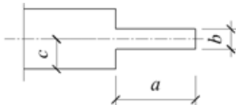
图 15.2.4-3 榫头示意图
