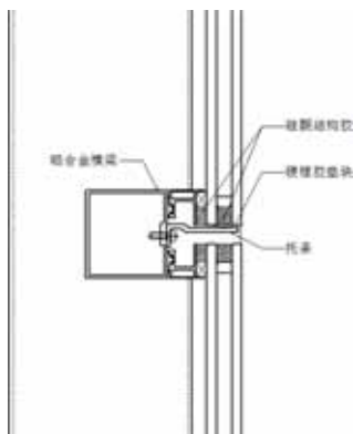
图 6-3 隐框托条构造示意一
