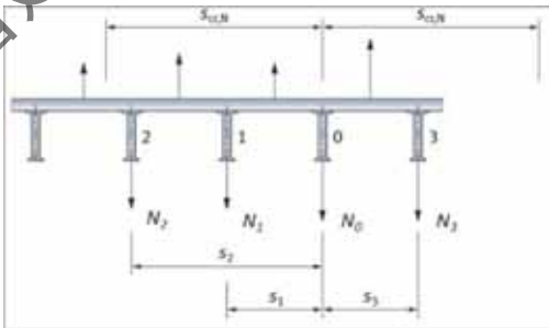
图 B. 3. 6 槽式预埋件受拉示意图
