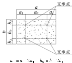
图 6.4.11-2 背栓支承时面板连接的计算边长 a_0 、 b_0
